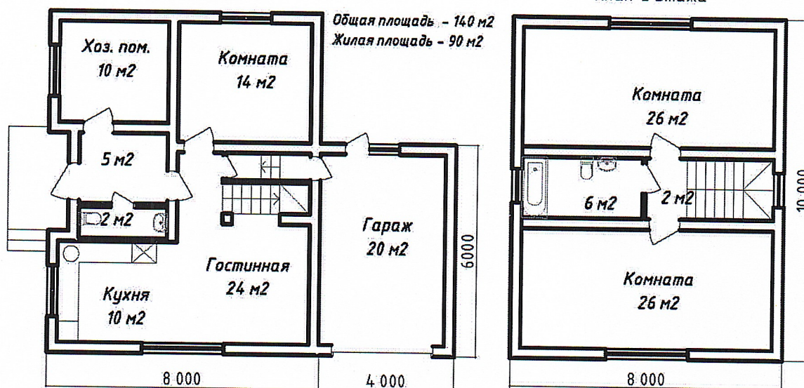
План 2 этажа
